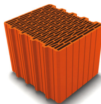
3. falazóelem-csoport vékonybordás, nagy üreges (PTH Klíma falazóelemek)
