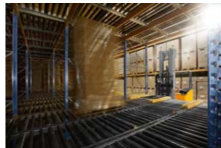
Görgős állvány
