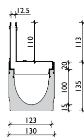
Részfolyóka rátét fedlap RSZ 12,5 C terh. oszt.
