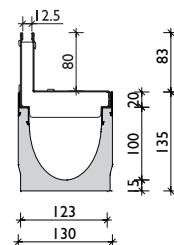
Részfolyóka rátét RSZ 12,5 C terh. oszt. B 125
