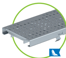
perforált rács horganyzott / rozsdamentes, Ø 6,0 mm A és C terh. oszt., NM 100-hoz C terh. oszt., NM 200-hoz
