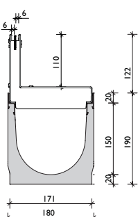
Résfolyóka rátét 2S, túsarokbiztos RSZ 2x6, C terhelési osztály
