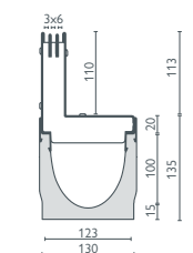
Részfolyóka rátét 3S, túsarokbiztos RSZ 3x6, C terh. oszt.y
