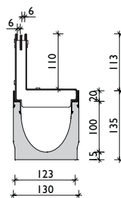
Részfolyóka rátét 2S, túsarokbiztos RSZ 2x6, C terh. oszt.
