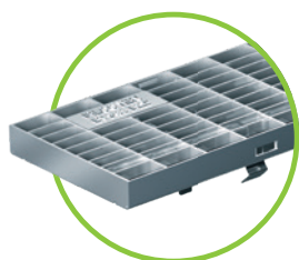
Hálós acél rács, B terh. oszt., horganyzott és C terh. oszt. horganyzott / rozsdamentes, RSZ 30/10, minden NM-hez
