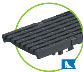
Hosszbordás öntöttvas rács, RSZ 29/6 szűk résszélesség, C terh. oszt., NM 100
