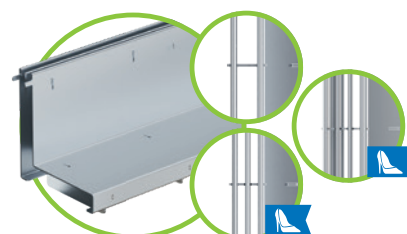
Részfolyóka rátét RSZ 12,5 mm, B terh. oszt., NM 100, V RSZ 12,5 mm, C terh. oszt. NM 100 / 150, V & E 2S, RSZ 2x6 mm, B terh. oszt. NM 100, E 2S, RSZ 2x6 mm, C terh. oszt. NM 100 / 150, V & E 3S, RSZ 3x6 mm, C terh. oszt. NM 100 / 150, E
